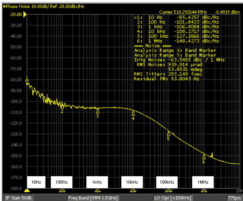
出力周波数 : 510.292857MHz
