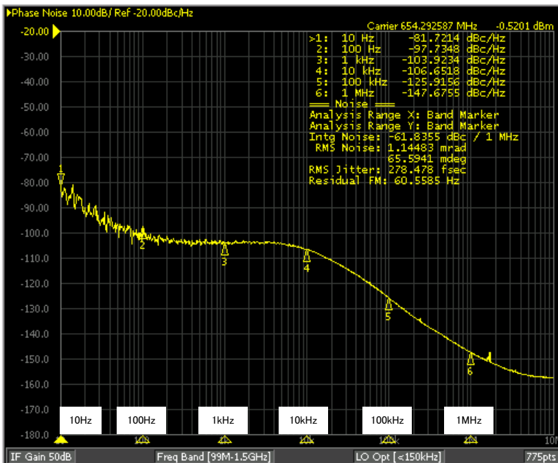
出力周波数 : 654.292857MHz
