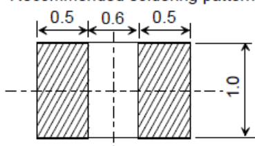
推奨はんだ付けパターン図 Recommended soldering pattern
