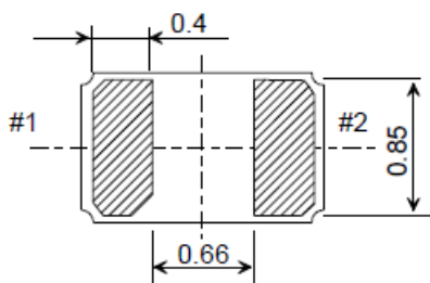
推奨はんだ付けパターン図 Recommended soldering pattern
